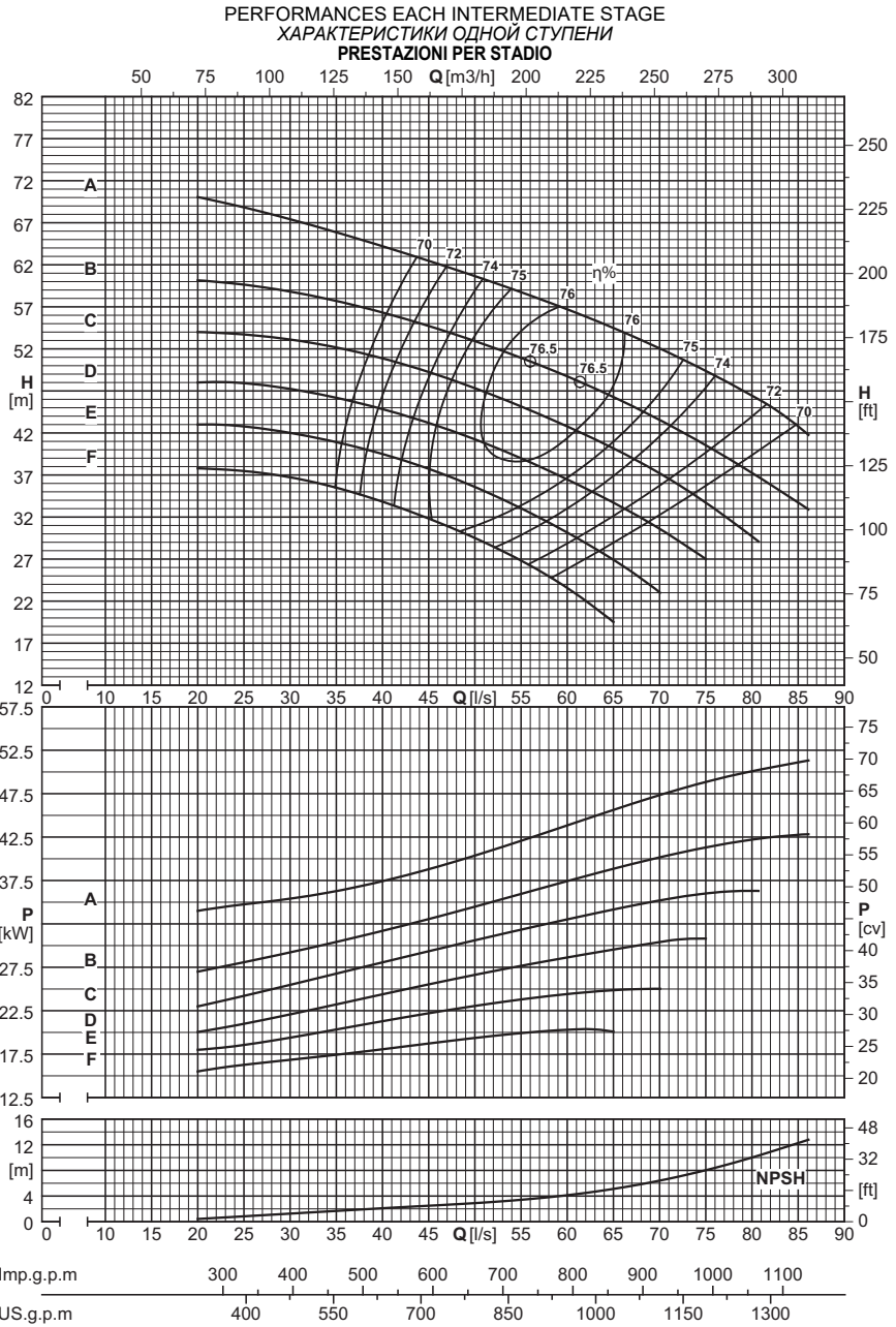
Capacity - Расход - Portata
