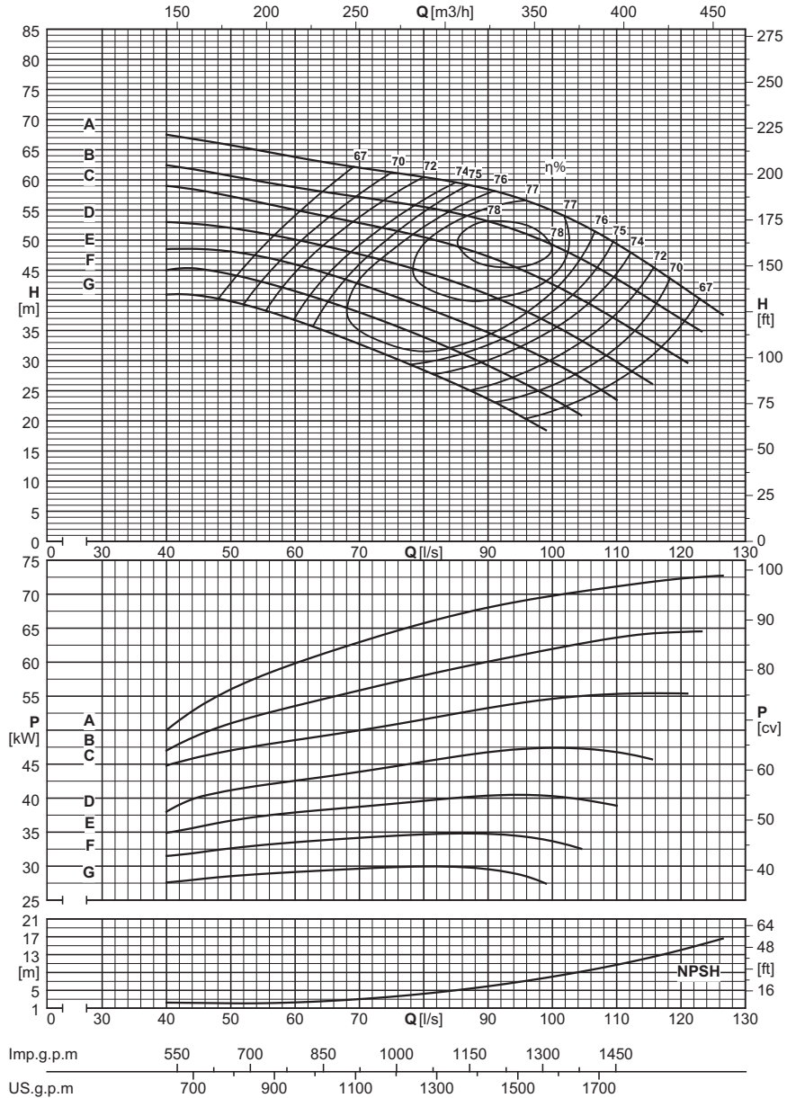
PERFORMANCES EACH INTERMEDIATE STAGE ХАРАКТЕРИСТИКИ ОДНОЙ СТУПЕНИ PRESTAZIONI PER STADIO
