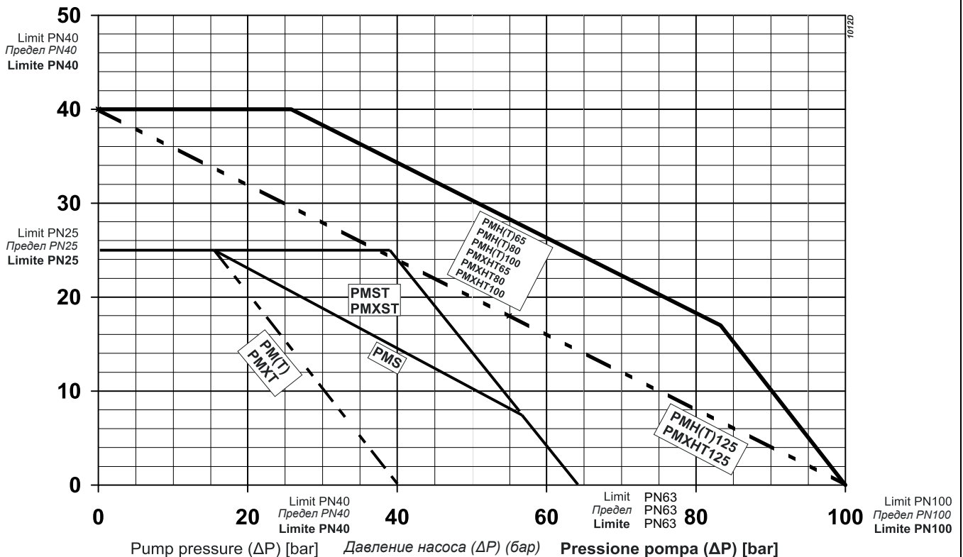
Test to ascertain the maximum pressure acting on the seals Проверка максимального давления, действующего на уплотнения Verifica della massima pressione agente sulle tenute
