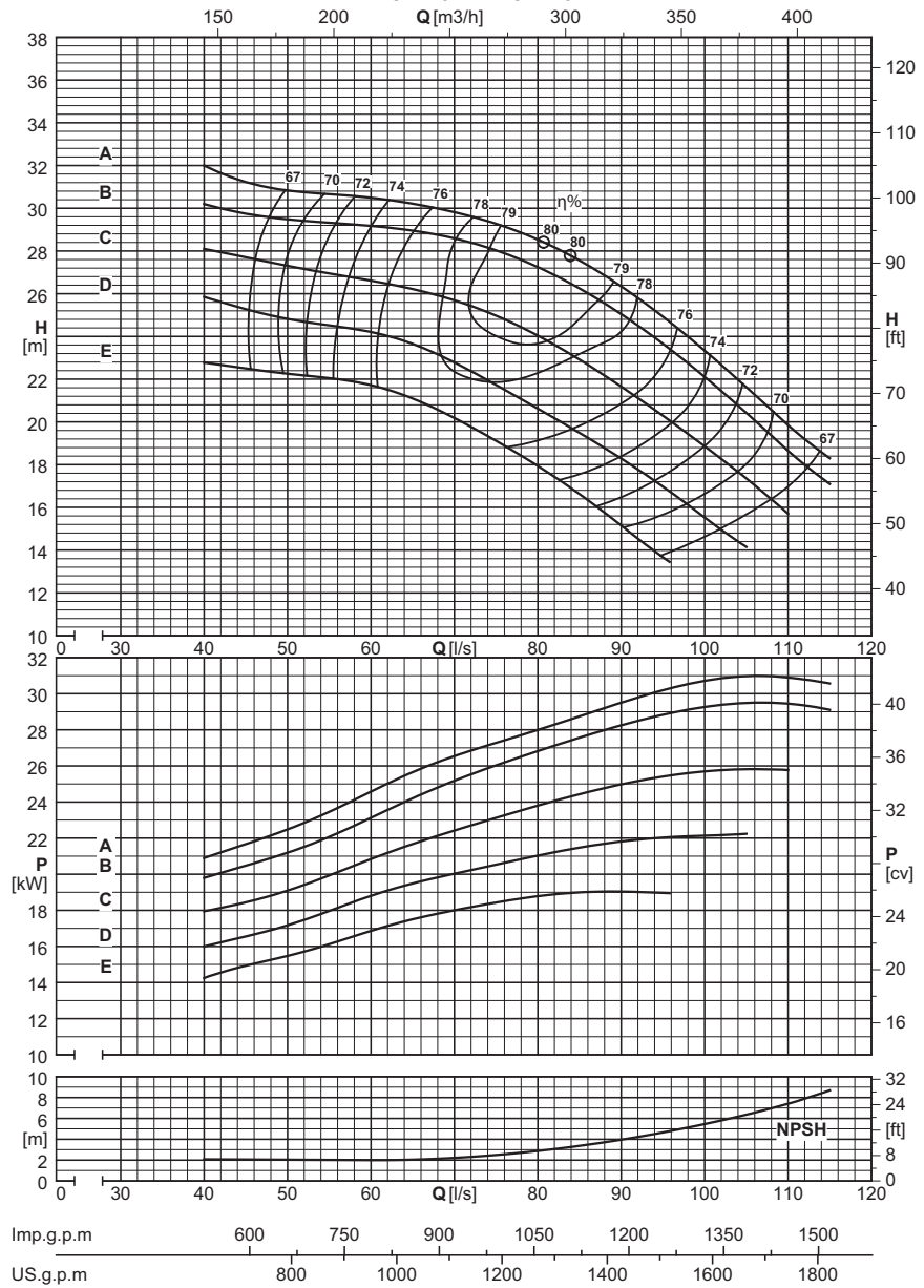
PERFORMANCES EACH INTERMEDIATE STAGE ХАРАКТЕРИСТИКИ ОДНОЙ СТУПЕНИ PRESTAZIONI PER STADIO
